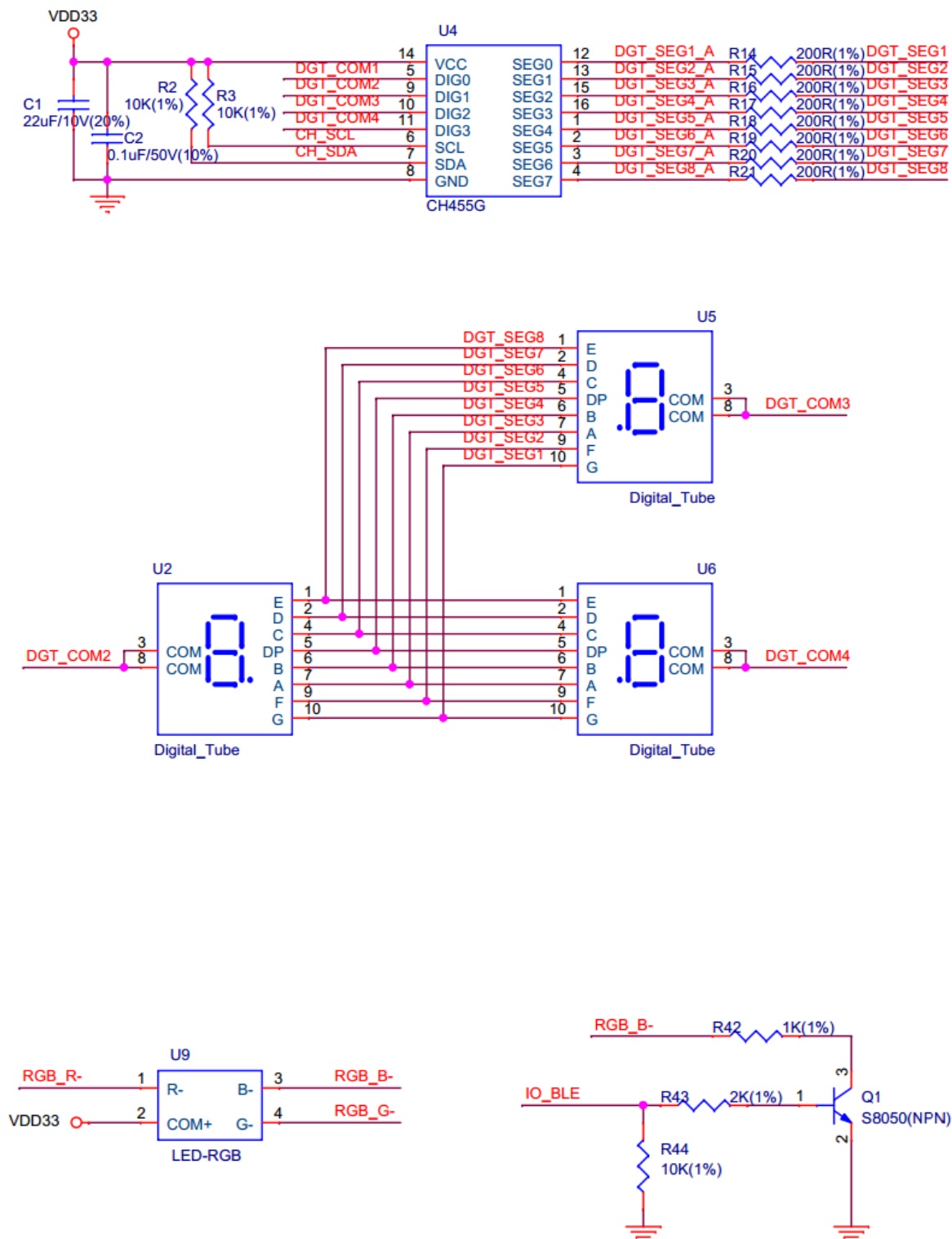
Fig. 10: Display Unit
